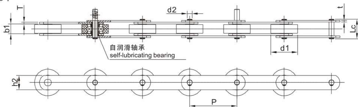
型式 II type II
