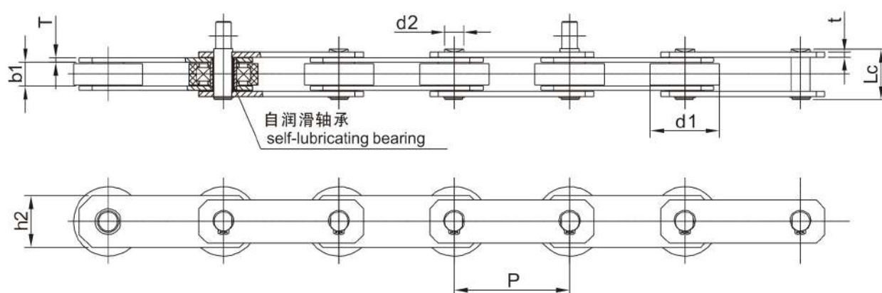
型式 II type II
